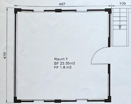
Erdgeschoss
