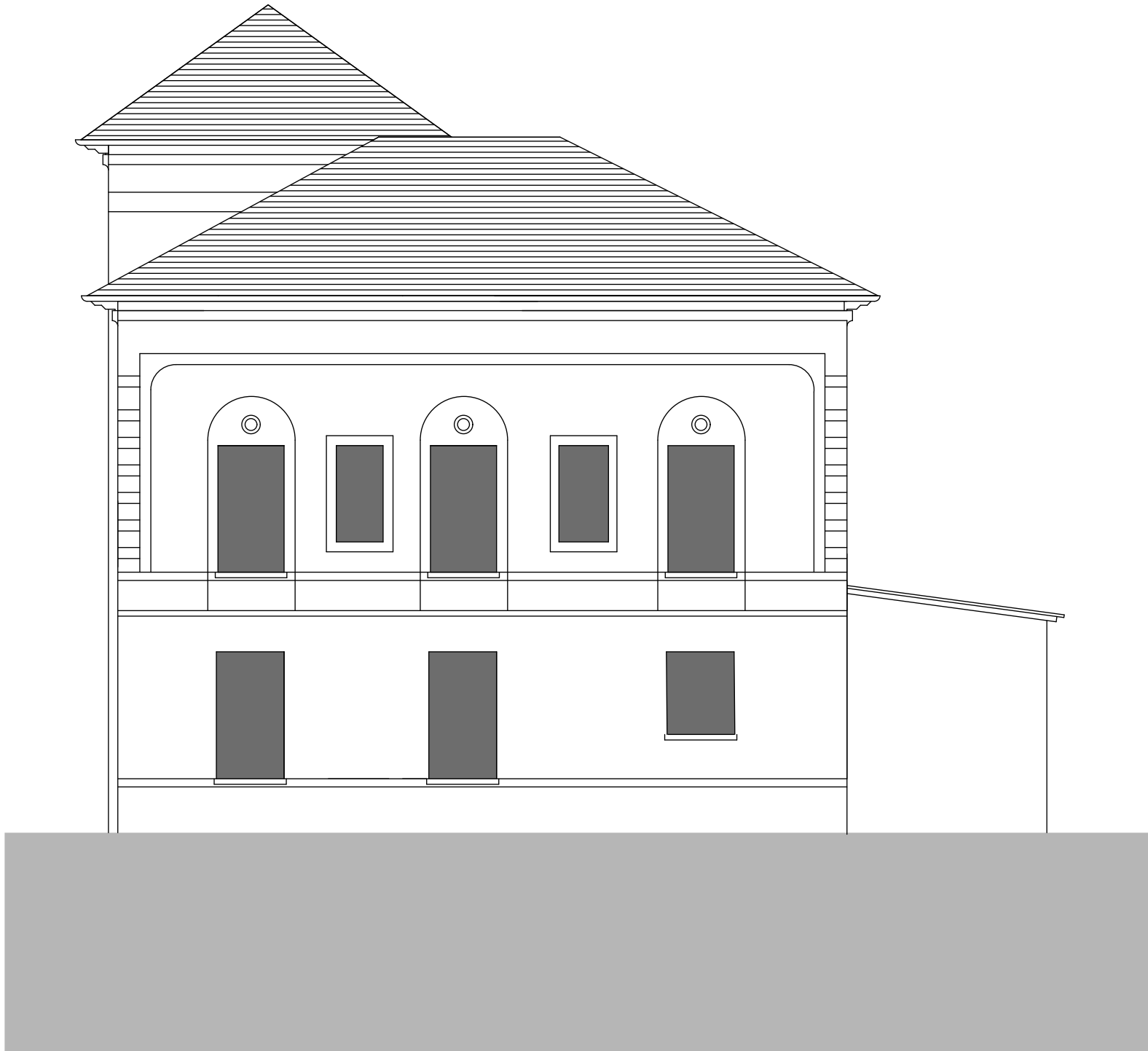
Facciata nord
