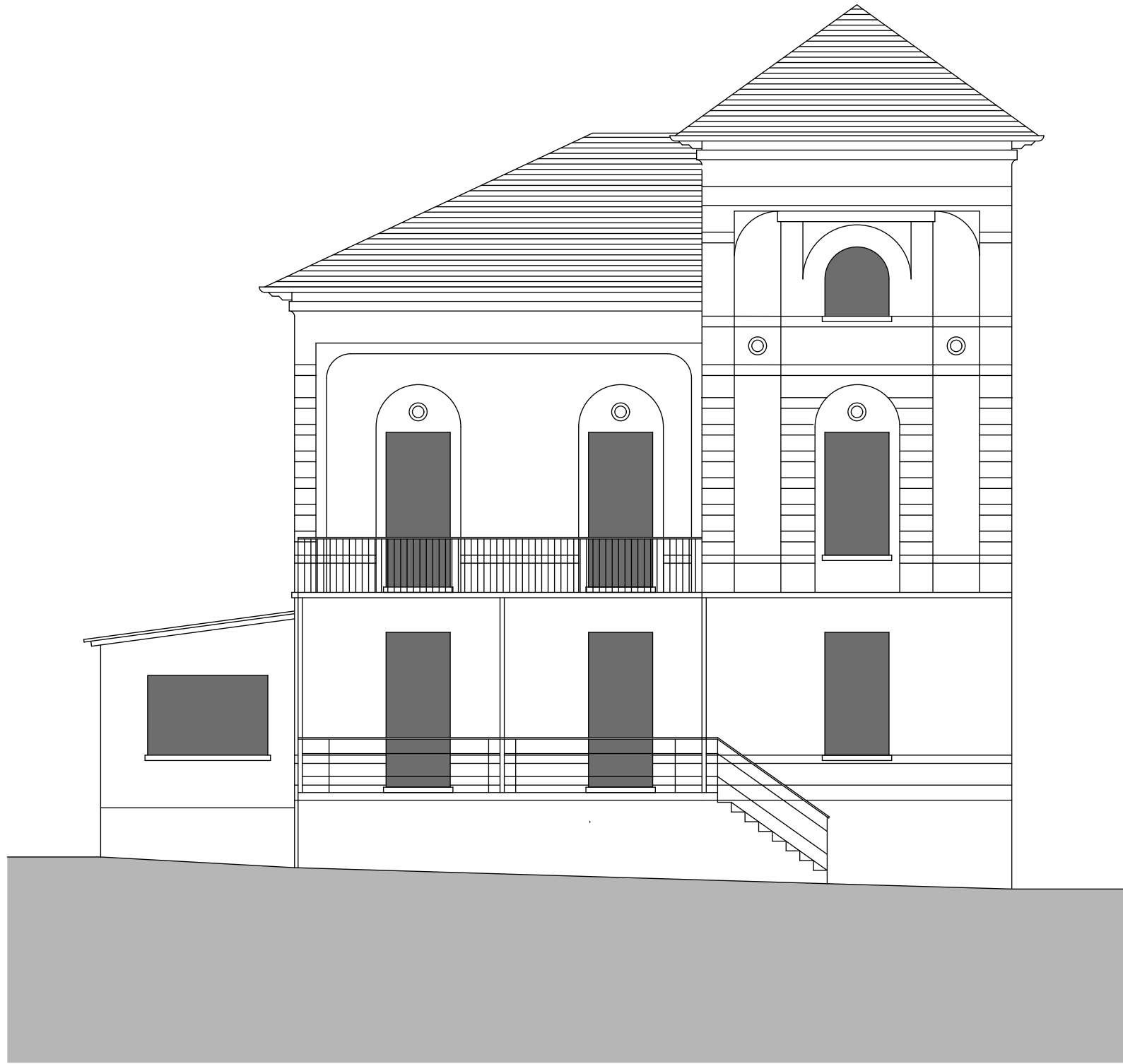
Facciata sud
