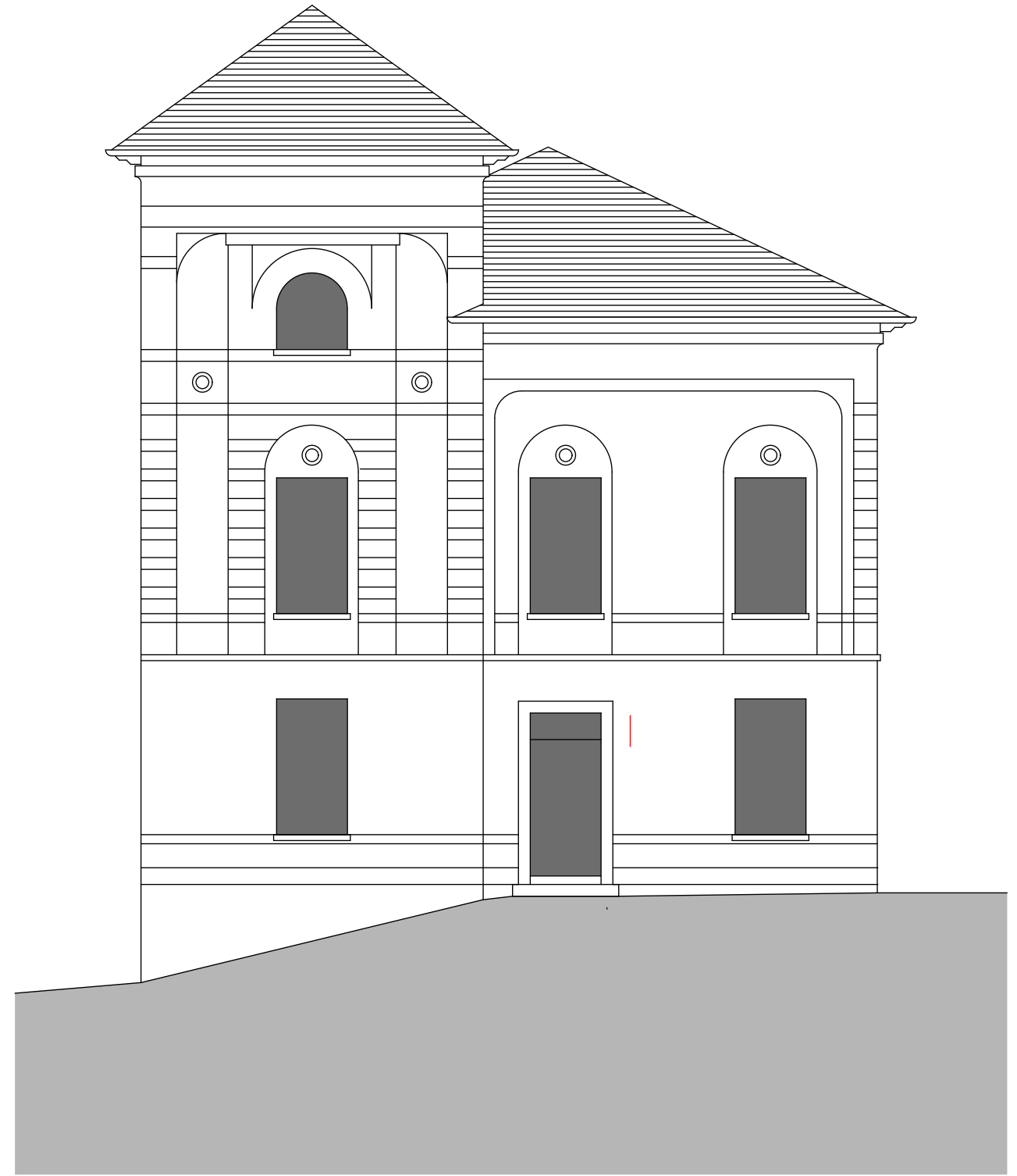
Facciata est
